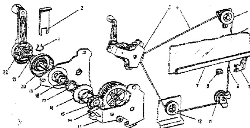
Fig. 8-14. Mecanismo de acionamento do vidro da porta: 1 - mola de retenção; 2 - dispositivo A.76034; 3 - mecanismo de acionamento do vidro; 4 - cabo; 5 - polia superior; 6 - vidro da porta; 7 - calha do vidro; 8 - fixador do cabo; 9 - capa do cabo; 10 - suporte da calha do vidro; 11 - polia inferior; 12 - polia tensora; 13 - suporte do mecanismo; 14 - tambor com engrenagem móvel; 15 - engrenagem motora; 16 - apoio do eixo; 17 - batente de arrasto da mola de frenagem; 18 - tampa do suporte; 19 - moldura; 20 - eixo da manivela; 22 - manivela.
