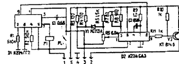
Fig. 7-27. Esquema do relé-disjuntor
