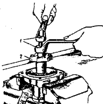
Fig. 2-63. Remoção do rotor: 1 - extrator; 2 - rotor.
