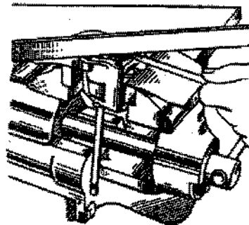
Fig. 2-70. Verificação das folgas axiais das engrenagens.
