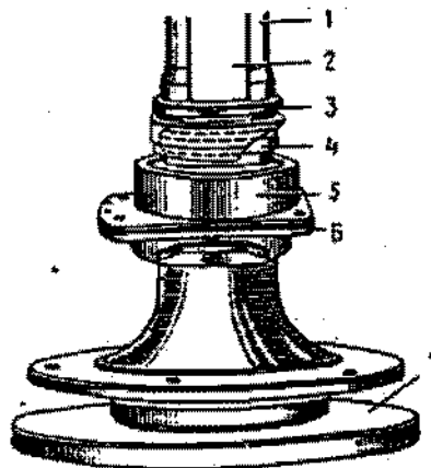
Fig. 3-56. Instalação do anel-trava: 1 - mandril; 2 - semi-árvore; 3 - aro; 4 - anel-trava; 5 - rolamento; 6 - placa de retenção do rolamento; 7 - anel de apoio.
