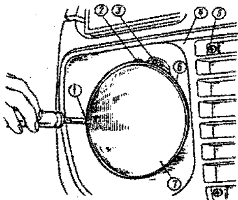
Fig. 7-24. Conjunto do farol: 1 - parafuso de ajuste horizontal; 2 - parafuso de ajuste vertical; 3 - parafuso de fixação do aro do farol; 4 - conjunto da grade dianteira e moldura dos faróis; 5 - parafuso de fixação da moldura; 6 - aro do farol; 7 - elemento ótico.
