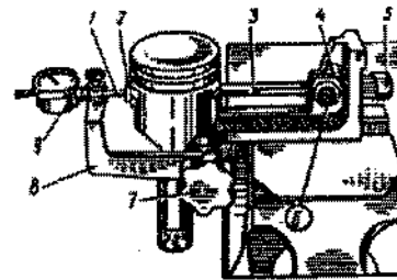
Fig. 2-33. Dispositivo para verificação da interferência de instalação: 1 - apalpador do micrômetro de dial; 2 - cabeça da haste em contato com o pino; 3 - haste roscaada com ranhura; 4 - base; 5 - porca da haste; 6 - fixador da ranhura da haste; 7 - manopla de fixação do suporte; 8 - suporte do micrômetro de dial; 9 - micrômetro de dial.
