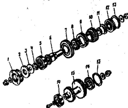
Fig. 3-35. Componentes das árvores propulsora e intermediária: 1 - flange; 2 - vedador; 3 - defletor de óleo; 4 - anel de encosto do rolamento; 5 - rolamento dianteiro; 6 - árvore propulsora; 7 - engrenagem de alta velocidade; 8 - cubo; 9 - luva; 10 - engrenagem de baixa velocidade; 11 - casquilho; 12 - rolamento traseiro; 13 - anel de ajuste do rolamento; 14 - rolamentos da árvore intermediária; 15 - árvore intermediária.
