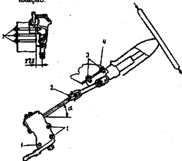
Fig. 5-4. Instalação do mecanismo da direção: 1 - porcas de fixação da caixa da direção; 2 - parafuso de fixação do terminal interior da árvore intermediária da coluna; 3 - parafusos de fixação do suporte; 4 - suporte da coluna da direção; 27,5 mm - distância do centro do alojamento do braço de comando até a superfície de apoio da caixa da direção, estando o braço na posição média.
