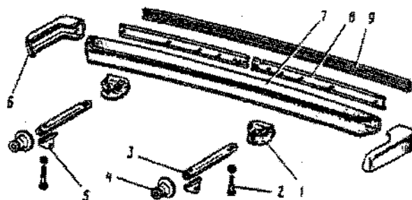
Fig. 8-22. Conjunto do pára-choque dianteiro: 1 - suporte; 2 - parafuso de fixação; 3 - suporte de fixação; 4 - vedação de borracha; 5 - aba de apoio do suporte; 6 - ponteiros plásticos; 7 - pára-choque; 8 - suporte da guarnição; 9 - guarnição.
