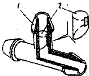
Fig. 8-26. Conexão "T" com estrangulador: 1 - conexão "T"; 2 - estrangulador.
