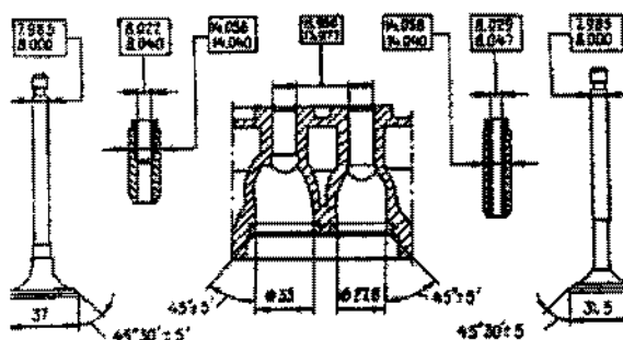
Fig. 2-40. Dimensões do cabeçote e válvulas
