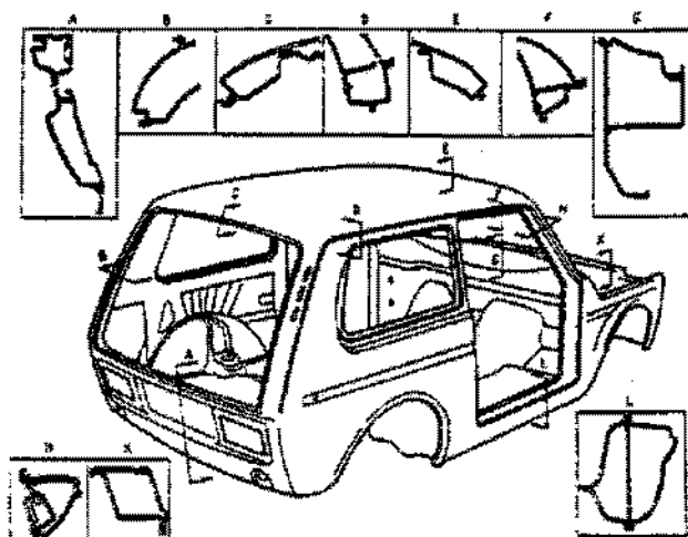
Fig. 8-3. Principais secções da carroceria
