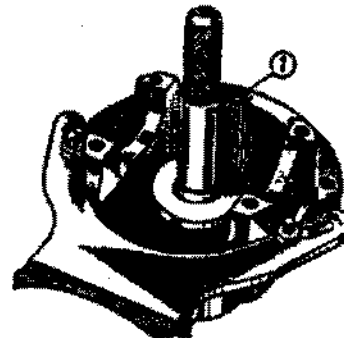
Fig. 3-64. Instalação da pista externa do rolamento traseiro do pinhão: 1 - mandril A.70171.
