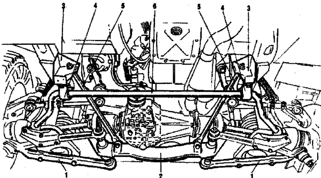
Fig. 4-6. Suspensão dianteira instalada no carro (vista por trás):
