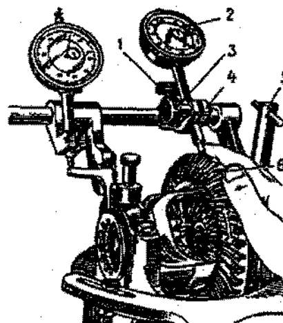
Fig. 3-72. Verificação da folga lateral de engrenamento: 1 - parafuso de fixação do suporte; 2 - micrômetro de dial; 3 - parafuso de fixação da haste do micrômetro; 4 - suporte do micrômetro de dial; 5 - parafuso de fixação; 6 - coroa.
