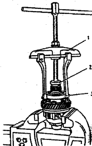
Figura 3-37 - Remoção dos rolamentos: 1 - extrator universal; 2 - apoio 67.7853-9559; 3 - rolamento.
