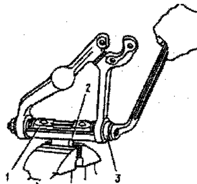
Fig. 4-11. Instalação das buchas do braço superior: 1 - eixo do braço; 2 - dispositivo 67.7853-9519; 3 - dispositivo A.74177/1.
