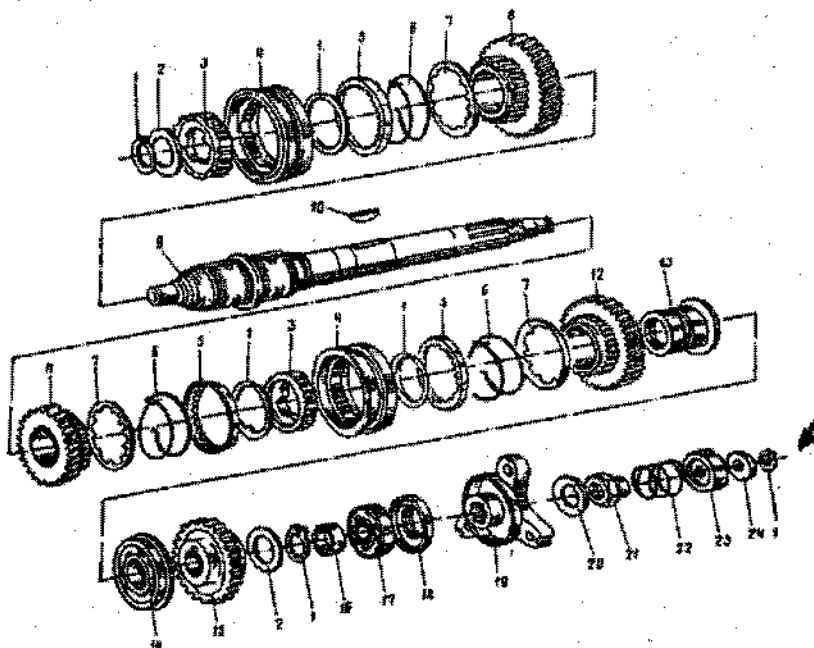
Fig. 3-25. Componentes da árvore secundária: 1 - anel de retenção; 2 - arruela elástica; 3 - cubo do sincronizador; 4 - luva do sincronizador; 5 - anel de bloqueio do sincronizador; 6 - mola do sincronizador; 7 - arruela; 8 - engrenagem de 3a.; 9 - árvore secundária; 10 - chaveta; 11 - engrenagem de 3a.; 12 - engrenagem de 1a.; 13 - casquilhos da engrenagem de 1a.; 14 - rolamento; 15 - engrenagem de ré; 16 - casquilho de encosto; 17 - rolamento traseiro; 18 - vedador; 19 - flange do acoplamento elástico; 20 - arruela de retenção; 21 - porta; 22 - mola de retenção; 23 - cubo de retenção; 24 - anel de centralização.
