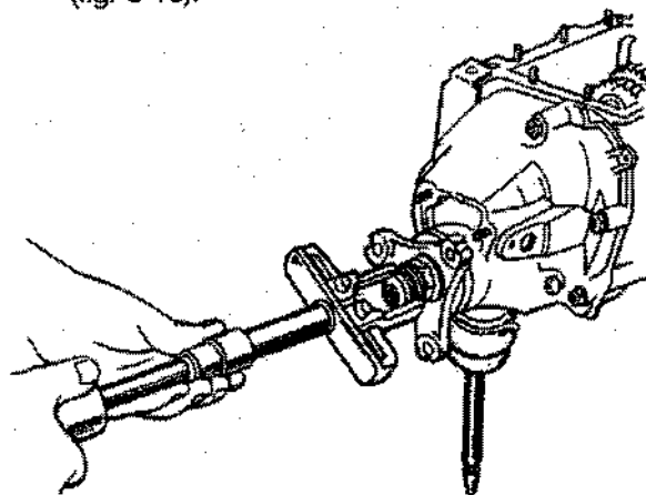
Fig. 3-15. Remoção do anel de centralização
