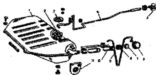
Fig. 2-79. Conjunto do tanque de combustível e tubulações: 1 - tanque de combustível; 2 - bóia medidora de nível; 3 - junta; 4 - tubulação de combustível; 5 - bomba de combustível; 6 - tampa do tanque; 7 - junta; 8 - conexão do tubo de enchimento; 9 - tubo de respiro; 10 - tubo de enchimento; 11 - moldura dos tubos de enchimento e de respiro.
