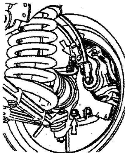
Fig. 6-14. Fixação do freio dianteiro: As setas indicam os parafusos de fixação do conjunto do freio.
