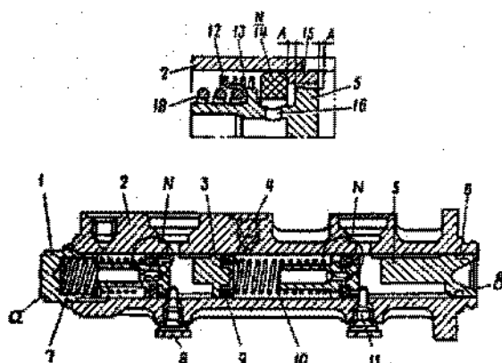
Fig. 6-10. Conjunto do cilindro mestre: 1 - tampão; 2 - corpo do cilindro; 3 - êmbolo de comando dos freios dianteiros; 4 - arruela; 5 - êmbolo de comando dos freios traseiros, e pressão adicional dos freios dianteiros; 6 - anel de vedação; 7 - mola de retorno dos êmbolos; 8, 11 - parafusos posicionadores dos êmbolos; 9, 14 - gaxetas dos êmbolos; 10 - mola de retorno dos êmbolos; 12 - prato da mola; 13 - mola de pressão da gaxeta; 15 - anel espaçador; 16 - orifício de admissão do fluido; A - orifício de compensação (folga entre a gaxeta 14, anel espaçador 15 e êmbolo 5).
