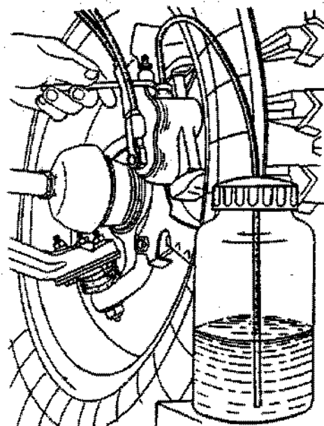
Fig. 6-8. Sangria do sistema hidráulico de freios
