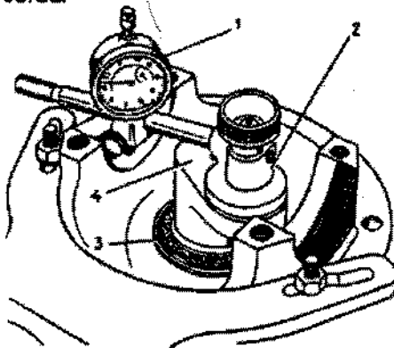
Fig. 3-65. Determinação da espessura do anel de ajuste: 1 - micrômetro de dial; 2 - dispositivo A.95690; 3 - rolamento traseiro do pinhão; 4 - bloco simulador A.70184.
