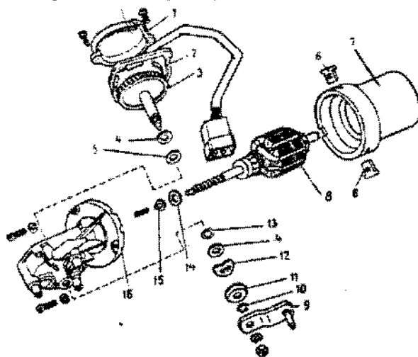
Fig. 7-31. Componentes do motor elétrico do limpador do pára-brisa: 1 - tampa; 2 - placa; 3 - engrenagem redutora; 4 - arruela de aço; 5 - arruela sintética; 6 - presilhas de fixação dos parafusos; 7 - carcaça; 8 - induzido; 9 - manivela; 10 - anel de retenção; 11 - capa de proteção; 12 - arruela elástica; 13 - anel de vedação; 14 - arruela de ajuste; 15 - centralizador; 16 - tampa.
