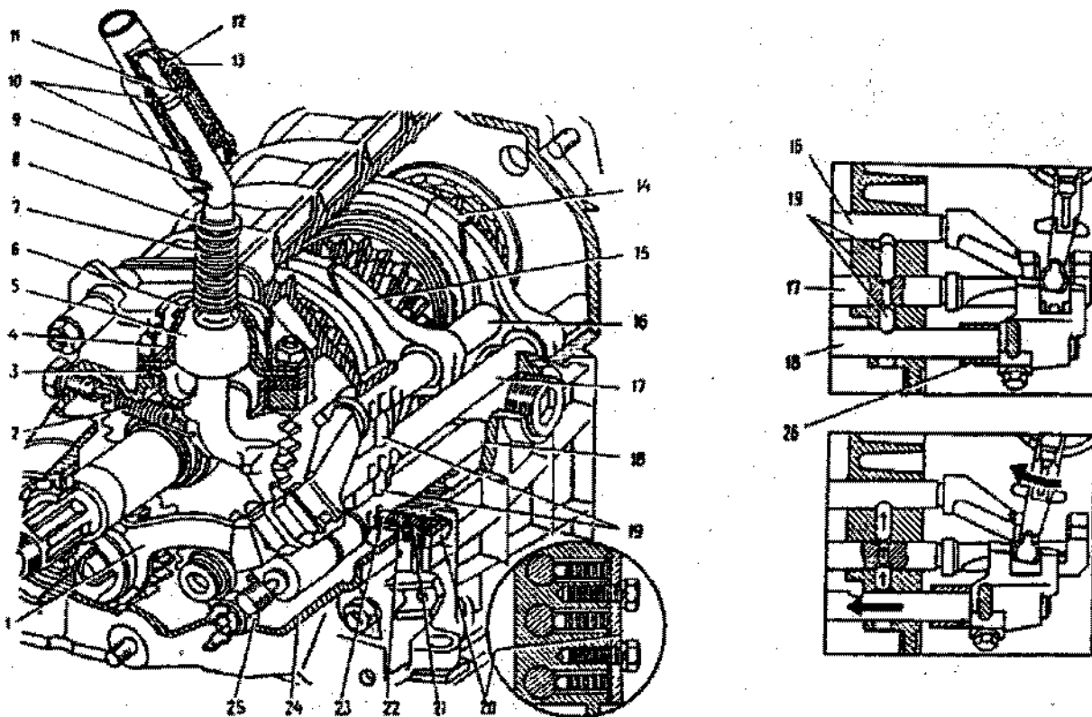
Fig. 3-20. Comandos de mudanças das marchas: 1 - garfo de conexão da ré; 2 - mola de retorno da alavanca; 3 - guia da rótula da alavanca; 4 - apoio esférico da rótula; 5 - alavanca de mudanças; 6 - arruela esférica; 7 - mola da alavanca; 8 - anel de retenção; 9 - bucha de bloqueio; 10 - buchas de borracha; 11 - espaçador; 12 - coxim de encosto; 13 - capa da alavanca de mudanças; 14 - garfo seletor de 3a. e 4a.; 15 - garfo seletor de 1a. e 2a.; 16 - haste deslizante de 1a. e 2a.; 17 - haste deslizante de 3a. e 4a.; 18 - haste deslizante da ré; 19 - cilindros bloqueadores; 20 - tampa de fixação das hastes deslizantes; 21 - casquilho; 22 - mola da esfera; 23 - esferas de retenção; 24 - tampa traseira; 25 - conector da lanterna da ré; 26 - espaçador da haste deslizante do garfo da ré.
