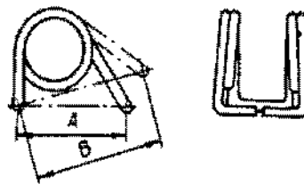
Fig. 2-50. Verificação da mola de alavanca: A - dimensão em estado livre; B - dimensão sob carga.
