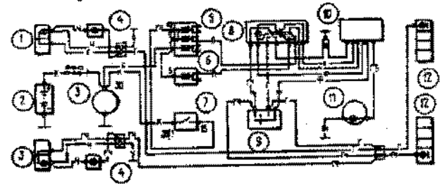
Fig. 7-26. Esquema do sistema de sinalização de advertência e indicadores direcionais: 1 - lanternas dianteiras; 2 - bateria; 3 - alternador; 4 - indicadores direcionais laterais; 5 - caixa de fusíveis principal; 6 - caixa de fusíveis suplementar; 7 - interruptor de ignição; 8 - interruptor da sinalização de advertência; 9 - comutador dos indicadores direcionais; 10 - relé-disjuntor da sinalização de advertência e indicadores direcionais; 11 - lâmpada indicadora dos indicadores direcionais; 12 - lanternas traseiras.
