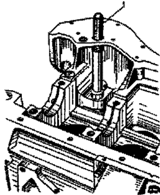
Fig. 2-73. Substituição do casquilho da engrenagem de acionamento da bomba de óleo: 1 - mandril A.60326/R.
