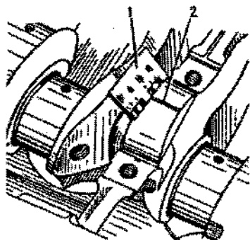
Fig. 2-37. Verificação da folga entre casquilho e munhão: 1 - escala do dispositivo de verificação; 2 - filete plástico de verificação.
