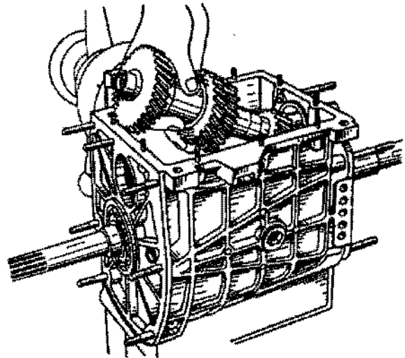
Fig. 3-19. Remoção da árvore intermediária
