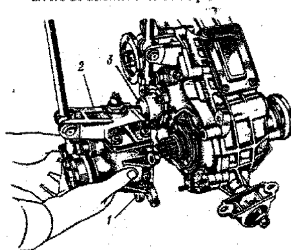
Fig. 3-33. Remoção do cárter do acionamento da tração dianteira: 1 - cárter; 2 - tampa do cárter; 3 - alojamento do acionamento do velocímetro.
