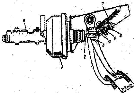
Fig. 6-3. Pedal do freio: 1 - servofreio; 2 - haste de acionamento; 3 - pedal do freio; 4 - batente do interruptor da luz de freio; 5 - porca do interruptor; 6 - interruptor da luz do freio; 7 - mola de retorno do pedal; 8 - cilindro mestre.
