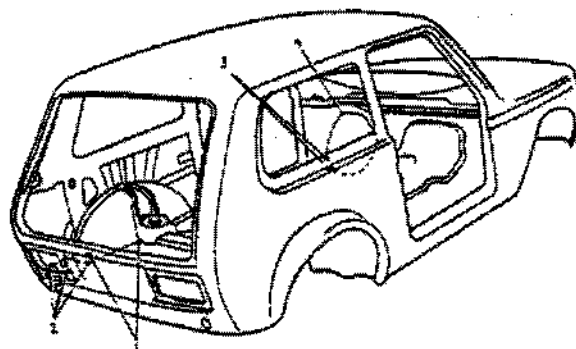
Fig. 8-11. Locais de aplicação da massa de calafetagem (vista pela parte traseira da carroceria): 1 - uniões do assoalho com arco da roda traseira; 2 - uniões soldadas angulares do assoalho com os arcos das rodas traseiras, laterais e painel traseiro; 3 - uniões angulares do assoalho com o painel de fogo; 4 - união angular do painel de fogo com o montante lateral dianteiro.
