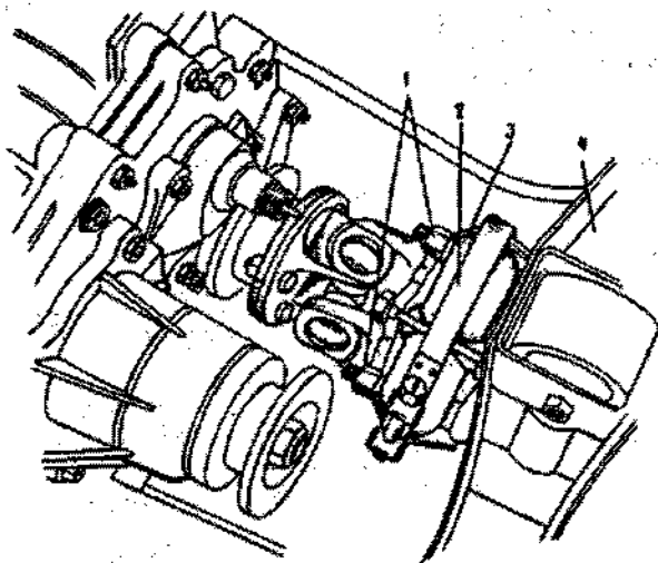
Fig. 3-12. Acoplamento elástico da união da árvore longitudinal com a caixa de mudanças: 1 - porcas de fixação do flange do cardã ao acoplamento elástico; 2 - braçadeira A.70025; 3 - acoplamento elástico; 4 - travessa do suporte traseiro do motor.
