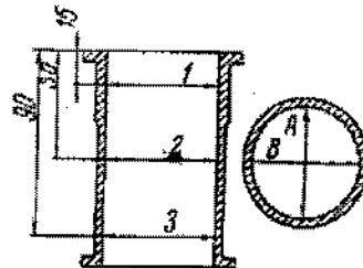
Fig. 3-23. Esquema de medição dos cilindros; A e B - sentido das medições; 1, 2 e 3 - número de medições.
