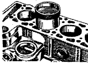
Fig. 2-15. Instalação dos conjuntos êmbolo/bielas nos cilindros
