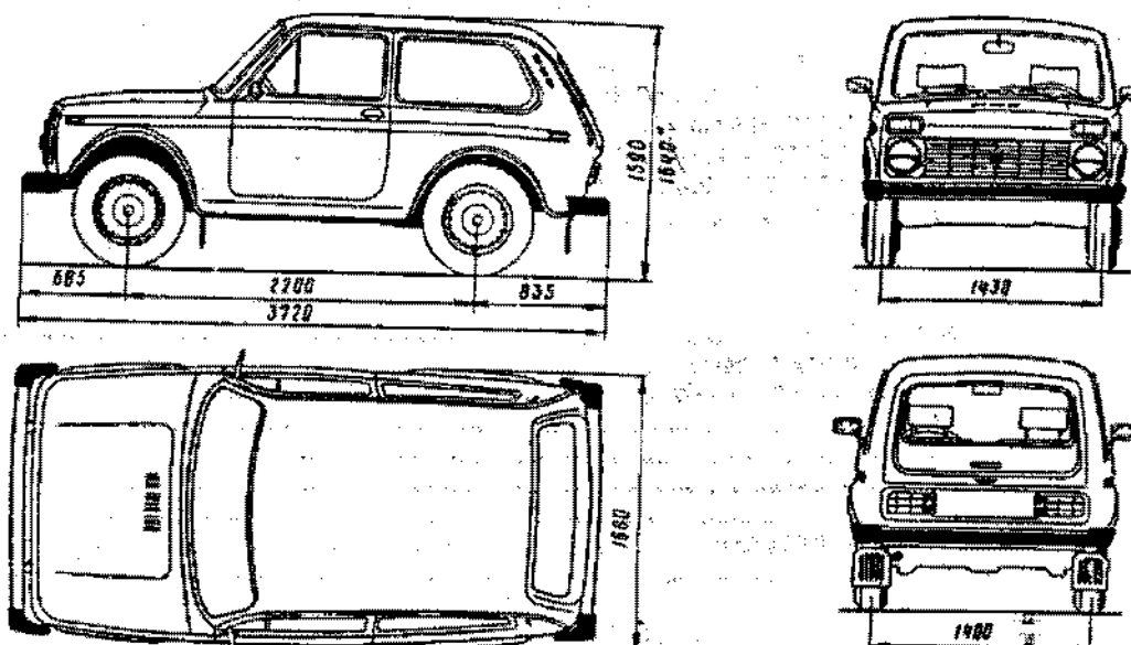
Fig. 1-1. Dimensões externas principais do veículo LADA 2121 (* altura sem carga)
