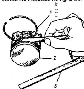
Fig. 2-28. Verificação da folga entre anéis e canaletas: 1 - anel de segmento; 2 - êmbolo; 3 - calibre de lâminas.
