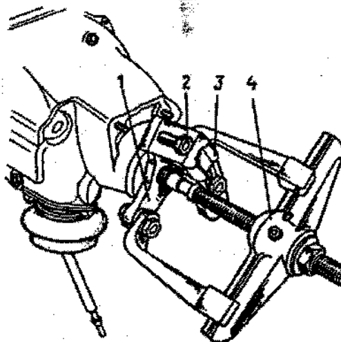
Fig. 3-16. Remoção do flange: 1 - flange do acoplamento elástico; 2 - parafusos de fixação do dispositivo ao flange; 3 - placa do extrator A.40005/3; 4 - extrator A.40005/3.
