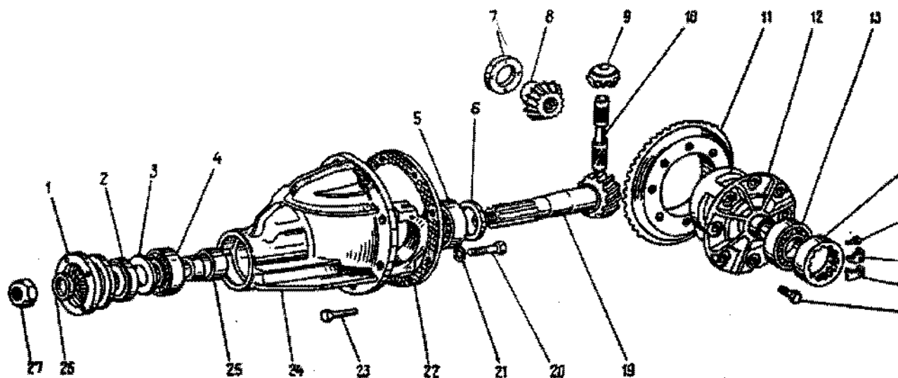
Fig. 3-63. Conjunto porta-diferencial: 1 - flange do pinhão; 2 - vedador; 3 - defletor de óleo; 4 - rolamento dianteiro; 5 - rolamento traseiro; 6 - anel de ajuste do pinhão; 7 - arruela de encaixe da planetária; 8 - planetária; 9 - satélite; 10 - eixo das satélites; 11 - coroa; 12 - caixa do diferencial; 13 - rolamento lateral da coroa; 14 - porca de ajuste; 15 - parafuso de fixação da placa de retenção; 16 - placa de retenção; 17 - placa de retenção; 18 - parafuso de fixação da coroa; 19 - pinhão; 20 - parafuso de fixação da capa; 21 - arruela elástica; 22 - junta; 23 - parafuso de fixação do porta-diferencial; 24 - porta-diferencial; 25 - bucha espaçadora; 26 - arruela plana; 27 - porca do flange do pinhão.
