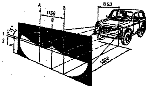
Fig. 7-25. Esquema para ajuste dos faróis
