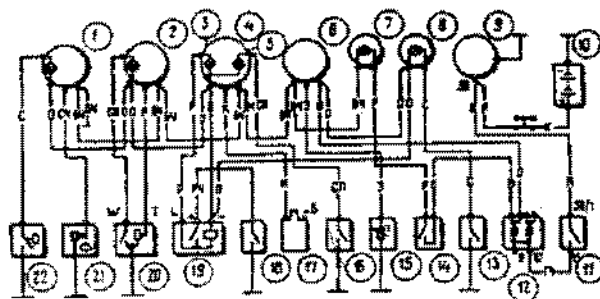
Fig. 7-36. Esquema de conexão dos instrumentos: 1 - indicador da pressão do óleo, com lâmpada indicadora de pressão baixa; 2 - indicador do nível do combustível, com lâmpada indicadora de reserva, 3 - lâmpada indicadora de freio de estacionamento acionado; 4 - tacômetro; 5 - lâmpada indicadora de afogador acionado; 6 - indicador da temperatura do líquido refrigerante; 7 - lâmpada indicadora do nível do fluido do freio; 8 - lâmpada indicadora do bloqueio do diferencial; 9 - alternador; 10 - bateria; 11 - interruptor da ignição; 12 - caixa de fusíveis; 13 - interruptor da luz de aviso do bloqueio do diferencial; 14 - bóia interruptora do nível baixo de fluido de freio; 15 - sensor do indicador da temperatura do líquido de arrefecimento do motor; 16 - interruptor da luz indicadora de afogador acionado; 17 - bobina da ignição; 18 - interruptor da luz indicadora de freio de estacionamento acionado; 19 - relé-disjuntor da luz indicadora do freio de estacionamento; 20 - sensor interruptor da luz de aviso de reserva de combustível; 21 - sensor do indicador da pressão do óleo; 22 - sensor da luz de advertência da pressão do óleo.
