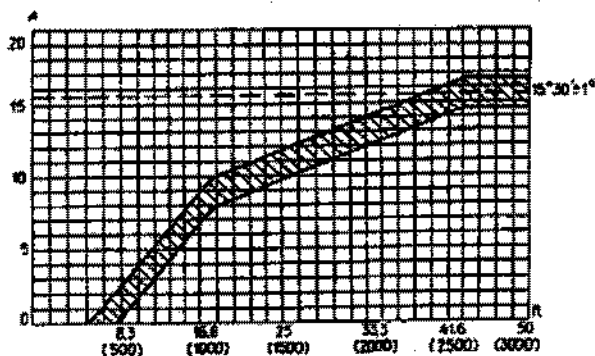
Fig. 7-19. Curva do avanço centrífugo do distribuidor: A - ângulo de avanço em graus; n - frequência de rotação do eixo do distribuidor, \text{s}^{-1} (rpm).
