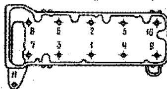
Fig. 2-16. Sequência de aperto dos parafusos do cabeçote
