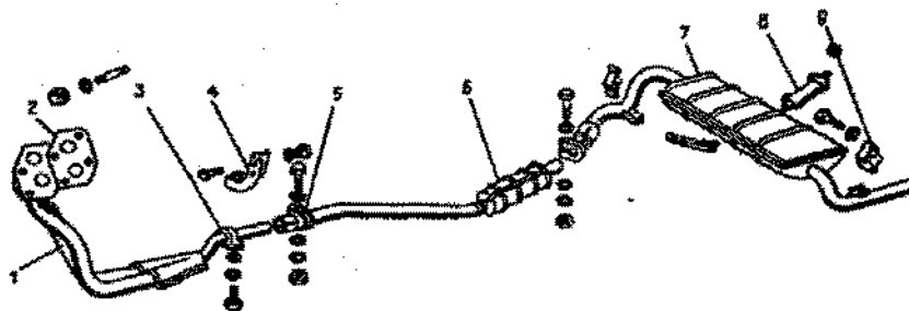
Fig. 2-95. Sistema de escapeamento: 1 - tubo de saída; 2 - junta; 3 - braçadeira do suporte da caixa de mudanças; 4 - suporte do conjunto do escapeamento; 5 - braçadeira de fixação dos conjuntos dos silenciadores; 6 - conjunto abafador; 7 - conjunto silenciador principal; 8 - correia de fixação do silenciador principal; 9 - coxim de sustentação do terminal do tubo.
