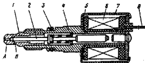
Fig. 2-92. Válvula de corte: 1 - gargulhante da marcha-lenta; 2 - agulhas; 3 - anel de vedação; 4 - corpo da válvula; 5 - placa de contato; 6 - bobina; 7 - armadura da bobina; 8 - terminal; A - orifício calibrado do gargulhante; B - orifício de saída do combustível.
