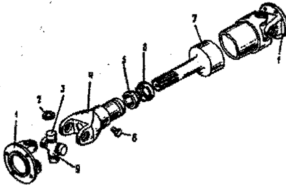
Fig. 3-45. Componentes da árvore longitudinal (cardã) dianteira: 1 - flange; 2 - anel de retenção; 3 - rolamento de agulhas; 4 - garfo deslizante; 5 - vedador; 6 - bucha; 7 - tubo do cardã; 8 - tampão; 9 - cruzeta.
