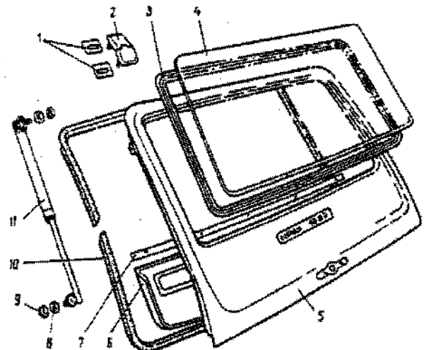
Fig. 8-18. Conjunto da porta traseira: 1 - junta; 2 - dobradiça; 3 - guarnição do vidro traseiro; 4 - vidro traseiro; 5 - porta; 6 - painel de acabamento interno da porta traseira; 7 - moldura de acabamento; 8 - arruela; 9 - porca de fixação do amortecedor; 10 - guarnição de vedação da abertura da porta; 11 - amortecedor a gás.
