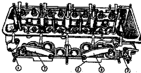
Fig. 2-52. Verificação da hermeticidade do cabeçote: 1, 2 e 4 - placas de vedação; 3 - base do dispositivo; 5 - flange com conexão para injeção de água.
