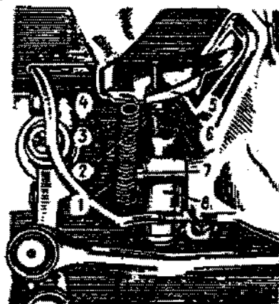
Fig. 3-11. Comandos da embreagem: 1 - mola de retorno; 2 - contraporta; 3 - porca de ajuste; 4 - contrapino; 5 - garfo da embreagem; 6 - haste; 7 - parafuso de fixação; 8 - cilindro atuador da embreagem.
