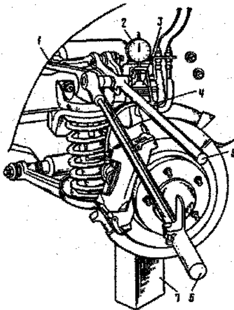
Fig. 4-3. Verificação da folga da articulação esférica: 1 - braço superior; 2 - micrômetro de dial; 3 - corpo da articulação esférica superior; 4 - suporte de fixação do micrômetro; 5 - braço; 6 - torquímetro; 7 - calço de madeira.
