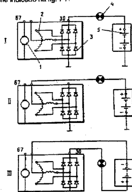
Fig. 7-7. Esquema de verificação dos diodos: I - verificação simultânea dos diodos positivos e negativos; II - verificação dos diodos negativos; III - verificação dos diodos positivos; 1 - rotor do alternador; 2 - enrolamento do estator; 3 - diodos; 4 - lâmpada de teste; 5 - bateria de teste.
