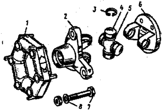
Fig. 3-46. Componentes do acoplamento elástico da árvore intermediária: 1 - acoplamento elástico; 2 - flange do acoplamento; 3 - anel de retenção; 4 - rolamento de agulhas; 5 - cruzeta; 6 - garfo de junta universal; 7 - parafuso de fixação do acoplamento elástico ao flange; 8 - arruela de balanceamento.
