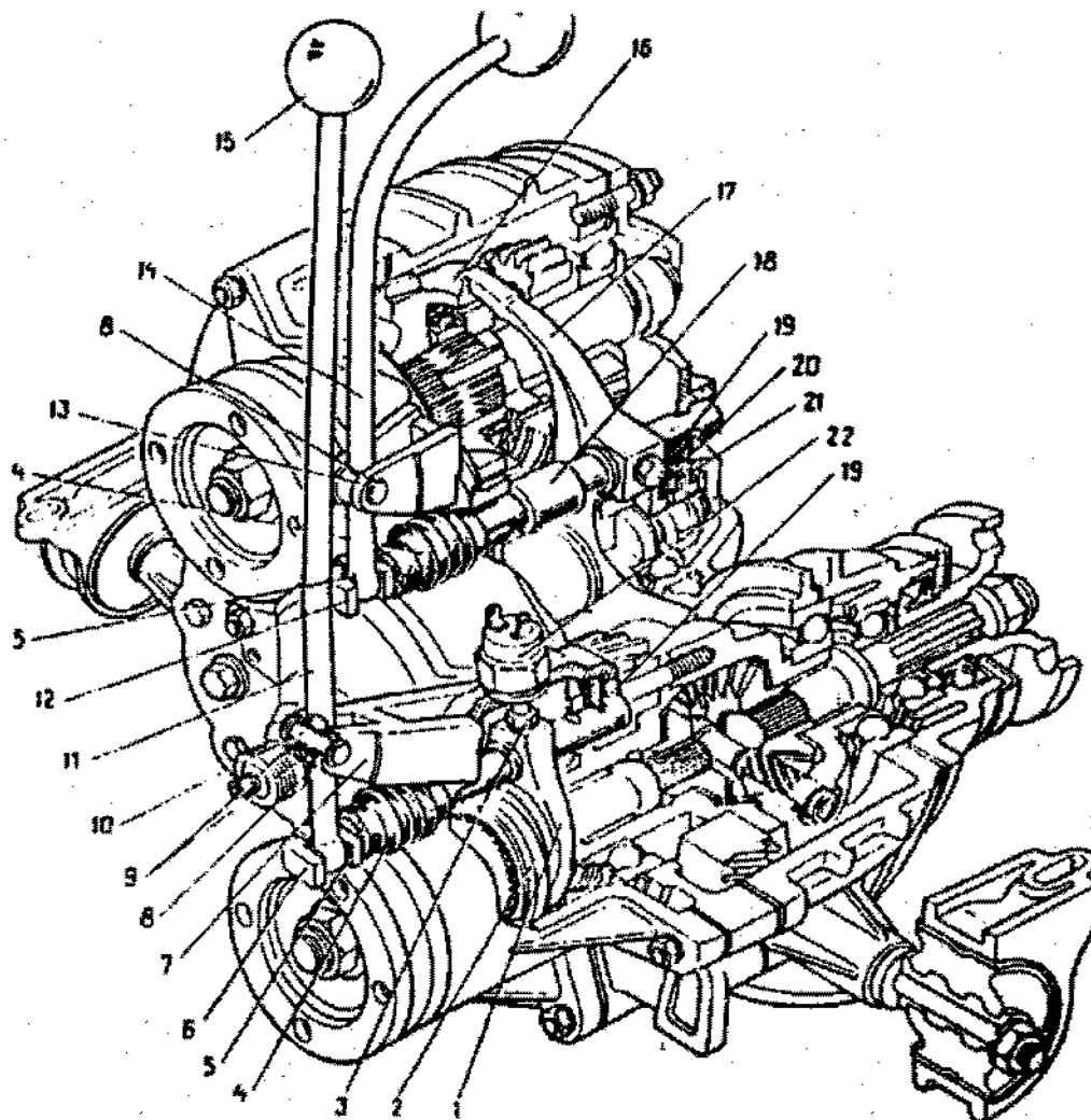
Fig. 3-30. Elementos de acionamento da caixa de transferência: 1 - garfo da luva do bloqueio do diferencial; 2 - luva do bloqueio do diferencial; 3 - parafuso de retenção do garfo; 4 - coifa de proteção da haste; 5 - mola da alavanca; 6 - haste da alavanca do bloqueio do diferencial; 7 - tampa do cárter do acionamento da tração traseira; 8 - arruela de retenção; 9 - casquilho do eixo da alavanca; 10 - eixo da alavanca; 11 - alavanca do bloqueio do diferencial; 12 - haste da alavanca de mudança de velocidades; 13 - suporte da alavanca de mudança de velocidades; 14 - alavanca de mudança de velocidades; 15 - manopla da alavanca; 16 - luva de mudança de velocidades; 17 - garfo da luva de mudança de velocidades; 18 - casquilho espaçador; 19 - esfera do mecanismo de retenção da haste; 20 - casquilho da mola do mecanismo de retenção da haste; 21 - mola do mecanismo de retenção da haste; 22 - interruptor da luz de aviso do bloqueio do diferencial.
