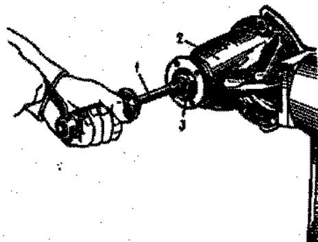
Fig. 3-70. Verificação do momento de resistência ao giro: 1 - dinamômetro 02.7812.9501; 2 - porta-diferencial; 3 - redutor.
