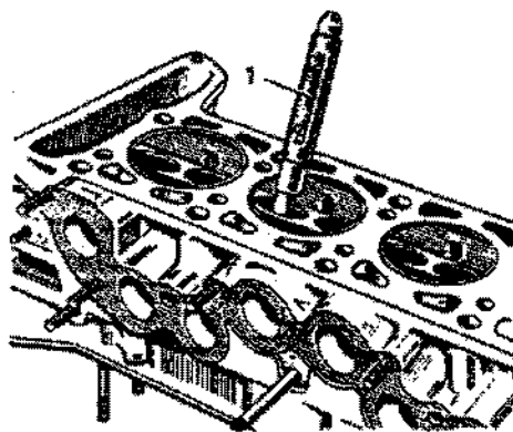
Fig. 2-47. Remoção dos guias das válvulas: 1 - mandril
