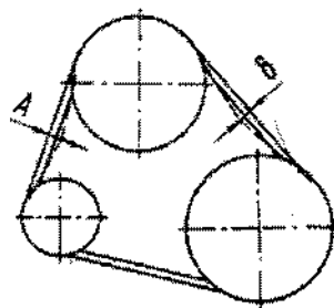
Fig. 2-61. Esquema para verificação da tensão da correia.
