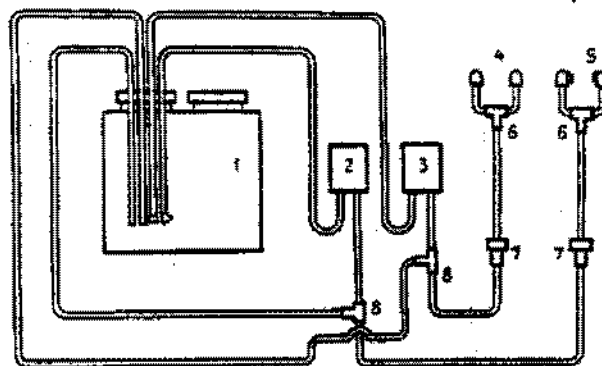
Fig. 8-25. Diagrama esquemático dos lavadores do pára-brisa e faróis: 1 - reservatório de líquido; 2 - bomba elétrica do lavador dos faróis; 3 - bomba elétrica do lavador do pára-brisa; 4 - ejetores do pára-brisa; 5 - ejetores dos faróis; 6 - conexões "T"; 7 - válvulas de retenção; 8 - conexões "T" com limitadores de vazão.
