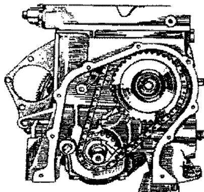
Fig. 2-17. Marcas de alinhamento da engrenagem e bloco
