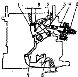
Fig. 2-94. Ajuste do dispositivo de partida: 1 - alavanca de acionamento do afoçador; 2 - borboleta do afoçador; 3 - vareta do dispositivo de partida; 4 - haste do dispositivo de partida; 5 - parafuso de ajuste; 6 - borboleta de aceleração primária; 7 - vareta de acionamento da borboleta.
