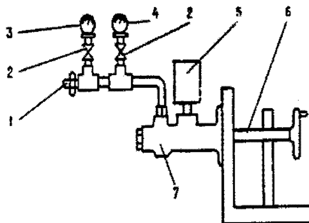
Fig. 3-9. Esquema de verificação da gaxeta dianteira: 1 - parafuso de sangria; 2 - registros; 3 - manômetro com divisão de 0,2 mPa (2 kgf/cm 2 ); 4 - manômetro com divisão de 0,005 mPa (0,05 kgf/cm 2 ); 5 - recipiente; 6 - manivela de acionamento do êmbolo; 7 - cilindro principal.
