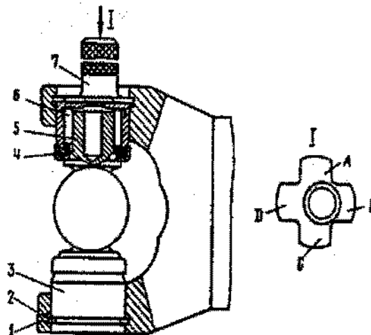
Fig. 3-47. Montagem da junta universal: 1 - garfo da junta universal; 2 - anel de retenção; 3 - corpo do rolamento; 4 - vedadores; 5 - espiga da cruzeta; 6 - agulha do rolamento; 7 - calibrador 41.8734-4092; A, B, C, D - lâminas do calibrador com espessura (em mm) 1,53; 1,56; 1,59; 1,62; I - vista superior do calibrador.
