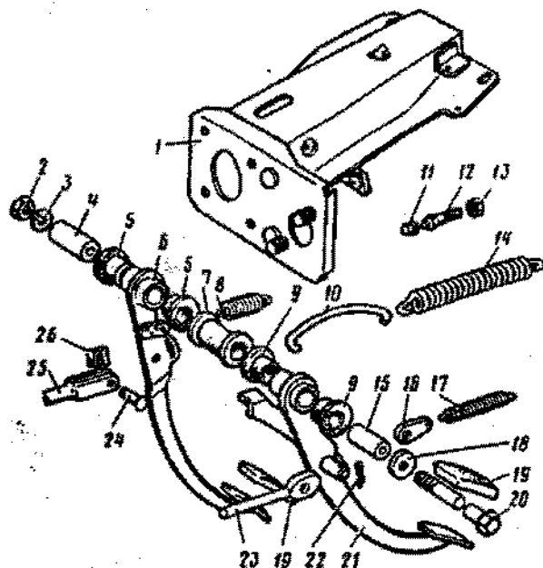
Fig. 8-9. Componentes do suporte dos pedais: 1 - suporte; 2 - porcas; 3 - arruela elástica; 4 - bucha interna do pedal do freio; 5 - buchas externas do pedal do freio; 6 - pedal do freio; 7 - espaçador; 8 - mola de retorno do pedal do freio; 9 - buchas externas do pedal da embreagem; 10 - gancho; 11 - capa protetora; 12 - parafuso limitador do pedal da embreagem; 13 - porca; 14 - mola de comando da embreagem; 15 - bucha interna do pedal da embreagem; 16 - suporte da mola; 17 - mola de retorno do pedal da embreagem; 18 - arruela; 19 - sapata do pedal; 20 - parafuso; 21 - pedal da embreagem; 22 - contrapino; 23 - haste de acionamento da embreagem; 24 - pino; 25 - haste de acionamento do servofreio; 26 - trava de retenção.
