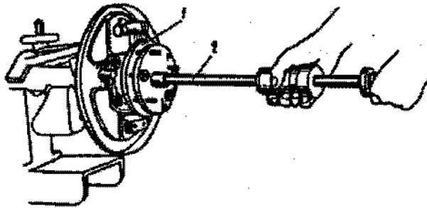
Fig. 3-49. Remoção da semi-árvore: 1 - semi-árvore; 2 - extrator 67.7823-9516.
