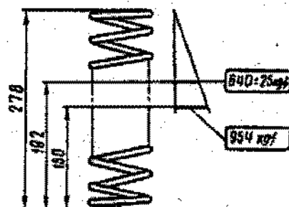
Fig. 4-9. Dados para verificação das molas
