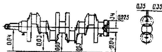
Fig. 2-36. Verificações da oscilação e coaxialidade.
