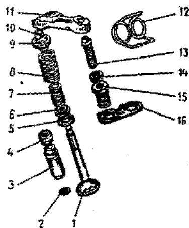
Fig. 2-41. Componentes do mecanismo das válvulas: 1 - válvula; 2 - anel retentor; 3 - guia; 4 - vedador da haste; 5 - arruela de apoio da mola externa; 6 - arruela de apoio da mola interna; 7 - mola interna; 8 - mola externa; 9 - prato da mola; 10 - travas; 11 - alavanca de acionamento da válvula; 12 - mola da alavanca; 13 - parafuso de ajuste; 14 - porca do parafuso de ajuste; 15 - casquilho do parafuso de ajuste; 16 - placa de retenção da mola da alavanca.
