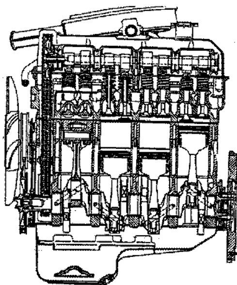
Fig. 2-1. Corte longitudinal do motor
