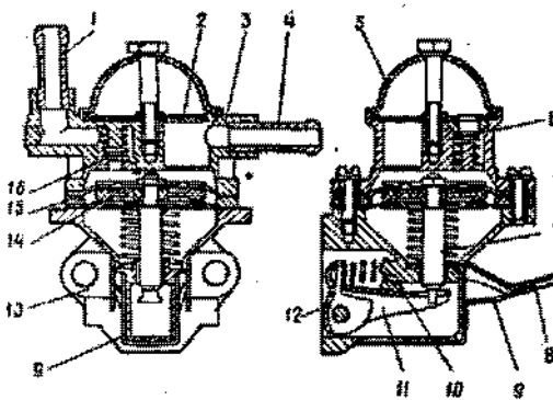
Fig. 2-77. Bomba de combustível: 1 - tubulação de pressão; 2 - filtro; 3 - carcaça; 4 - tubulação de aspiração; 5 - tampa; 6 - válvula de aspiração; 7 - haste; 8 - alavanca de alimentação manual de combustível; 9 - mola; 10 - excêntrico de acionamento; 11 - balancim; 12 - alavanca mecânica de alimentação de combustível; 13 - tampa inferior; 14 - junta espaçadora interna; 15 - junta espaçadora externa; 16 - válvula de pressão.
