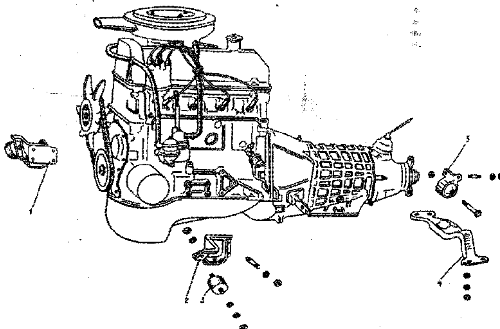
Fig. 2-3. Fixação do motor: 1 - suporte direito do motor com eixo; 2 - suporte esquerdo do motor; 3 - eixo; 4 - travessa de fixação traseira do motor; 5 - suporte traseiro do motor com apoio.
