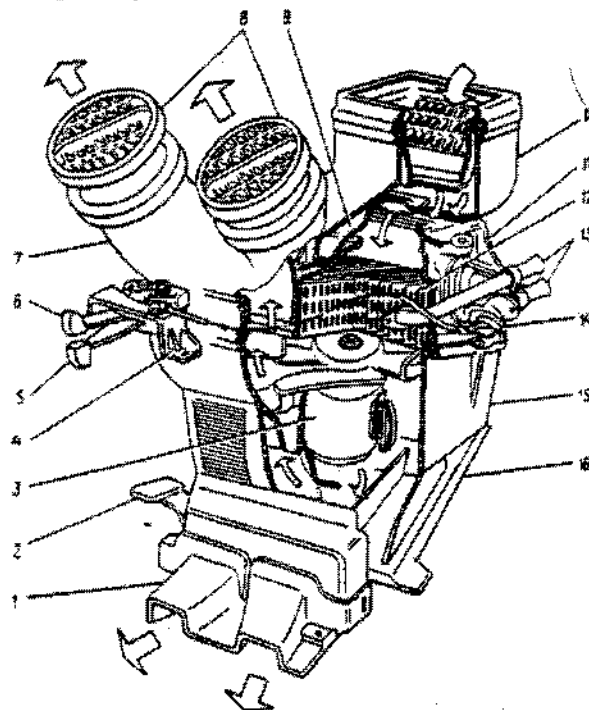
Fig. 8-33. Caixa da ventilação: 1 - duto de ar para ventilação inferior; 2 - alavanca de controle da distribuição do ar; 3 - ventilador elétrico; 4 - suporte das alavancas de comando; 5 - alavanca de comando do fluxo de ar; 6 - alavanca de controle da temperatura; 7 - tubos das grades de ventilação; 8 - grades direcionadoras; 9 - tampa do fluxo de ar; 10 - caixa do fluxo de ar; 11 - carcaça do radiador do aquecedor; 12 - radiador do aquecedor; 13 - tubos de alimentação e retorno do líquido de arrefecimento; 14 - motor elétrico; 15 - carcaça do ventilador; 16 - tampa de distribuição do ar.
