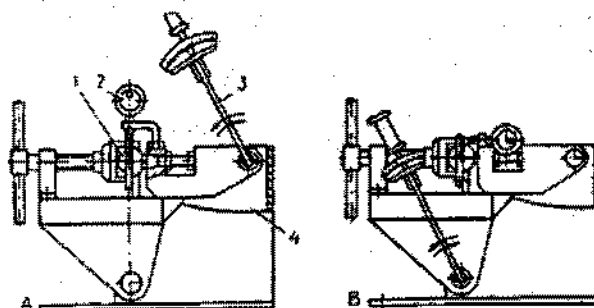
Fig. 4-8. Verificação da articulação esférica: 1 - articulação esférica; 2 - micrômetro de dial; 3 - torquímetro; 4 - dispositivo 02.8701-9502; A - esquema de verificação da folga radial; B - esquema de verificação da folga axial.
