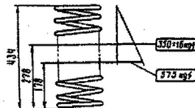
Fig. 4-17. Dados para verificação das molas
