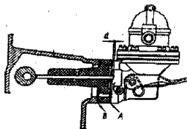
Fig. 2-78. Esquema para instalação da bomba de combustível: A - junta de espessura 0,27 - 0,33 mm; B - junta de espessura 0,70 - 0,80 mm; d - saliência do acionador.
