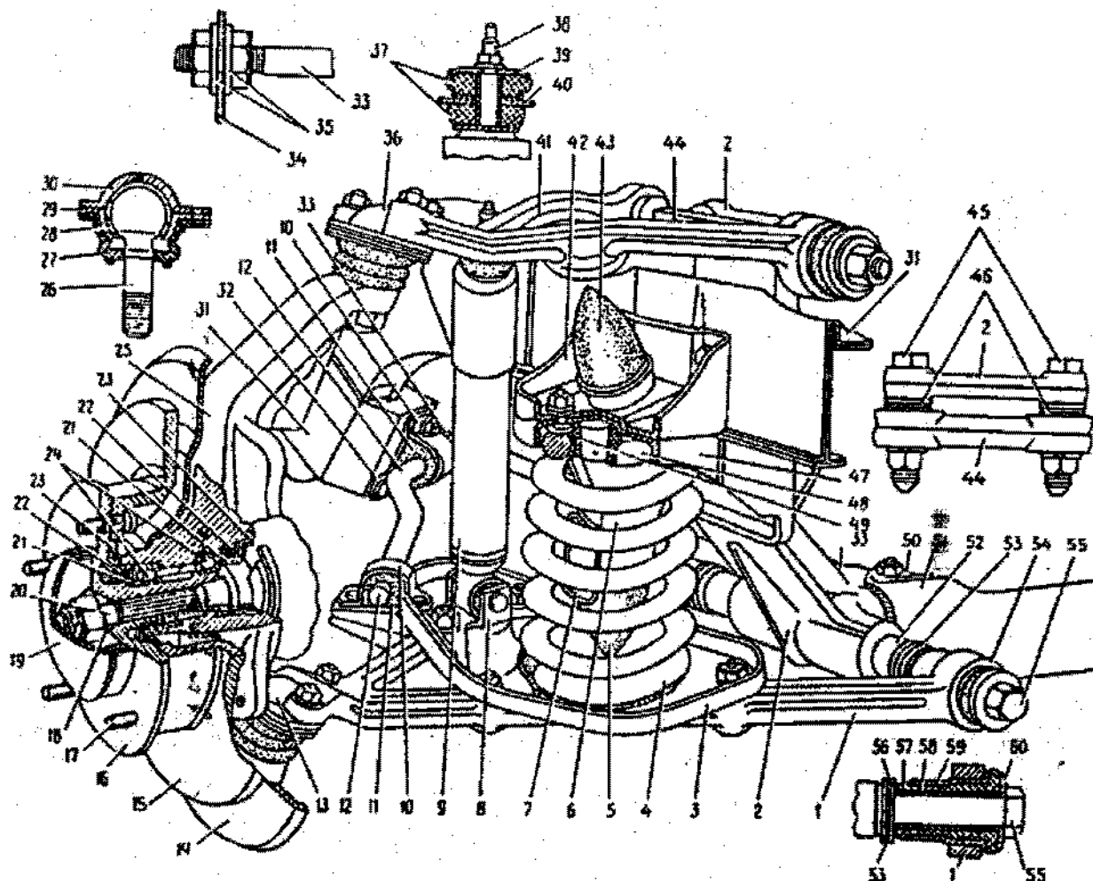
Fig. 4-1. Suspensão dianteira: 1 - braço inferior; 2 - suporte da travessa; 3 - suporte inferior da mola da suspensão; 4 - mola da suspensão; 5 - batente; 6 - suporte do batente; 7 - limitador de curso; 8 - suporte inferior de fixação do amortecedor; 9 - amortecedor; 10 - braçadeira de fixação da barra estabilizadora; 11 - isolador de borracha; 12 - barra estabilizadora; 13 - articulação esférica inferior; 14 - placa protetora do freio dianteiro; 15 - disco de freio; 16 - cubo da roda; 17 - prisioneiro de fixação do disco do freio e roda; 18 - casquilho cônico; 19 - calota; 20 - extremidade da ponta de eixo; 21 - anel do vedador; 22 - vedador; 23 - anel defletor de pó; 24 - rolamentos do cubo da roda; 25 - suporte da ponta de eixo; 26 - pino da articulação esférica; 27 - coifa; 28 - bucha; 29 - aro do casquilho da coifa; 30 - corpo do pino da articulação esférica; 31 - placa de fixação da barra estabilizadora; 32 - suporte da carroceria; 33 - tirante; 34 - suporte de fixação do tirante; 35 - arruelas; 36 - articulação esférica superior; 37 - isoladores de borracha da haste superior do amortecedor; 38 - haste do amortecedor; 39 - arruela; 40 - suporte de fixação do amortecedor; 41 - braço superior do amortecedor; 42 - suporte do batente; 43 - batente da suspensão; 44 - eixo do braço superior; 45 - parafusos de fixação do eixo do braço superior; 46 - arruelas de ajuste; 47 - apoio superior da mola da suspensão; 48 - isolador do apoio superior da mola; 49 - junta da mola; 50 - suporte de fixação do tirante à travessa; 51 - travessa da suspensão dianteira; 52 - bucha do eixo do braço inferior; 53 - arruelas de ajuste do braço inferior; 54 - articulação isolada do braço inferior; 55 - eixo do braço inferior da suspensão; 56 - arruela de apoio; 57 - isolador de borracha da articulação inferior; 58 - bucha interna da articulação; 59 - bucha externa da articulação; 60 - arruela de apoio da articulação.
