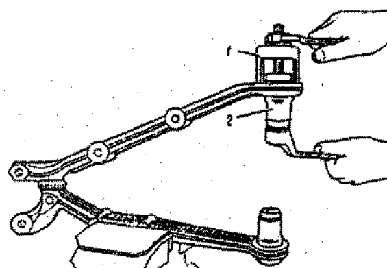
Fig. 4-12. Remoção da bucha isoladora do braço inferior: 1 - dispositivo 67.7823-9517; 2 - bucha isoladora.
