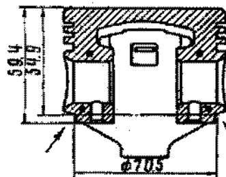
Fig. 2-30. Esquema para remoção de material do êmbolo
