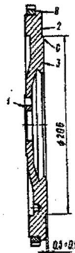
Fig. 2-38 - Volante: 1 - superfície de contato com o flange da árvore de manivelas; 2 - superfície de fixação do prato da embreagem; 3 - superfície de trabalho do disco; B - ponto de verificação da oscilação da superfície 2; C - ponto de verificação da oscilação da superfície 3.
