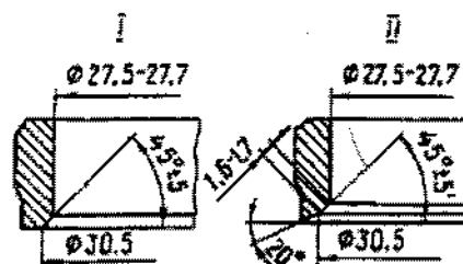
Fig. 2-44. Ângulos de assentamento das válvulas de escapamento: I - assento novo; II - após reparo.
