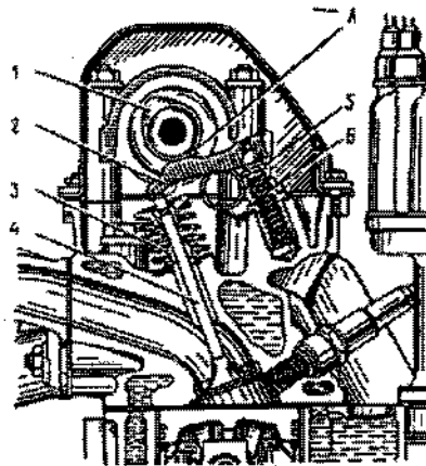
Fig. 2-54. Vista em corte do sistema de acionamento das válvulas: 1 - árvore de comando das válvulas; 2 - alavanca da válvula; 3 - vedador da haste; 4 - válvula de admissão; 5 - parafuso do ajuste; 6 - contraporca; A - folga entre alavanca e came.
