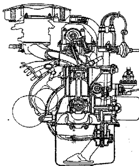
Fig. 2-2. Corte transversal do motor
