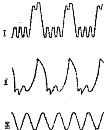
Fig. 7-6. Tipos de curva de tensão retificada do alternador: I - alternador em bom estado; II - diodo danificado; III - circuito dos diodos (enrolamento do estator) interrompido.
