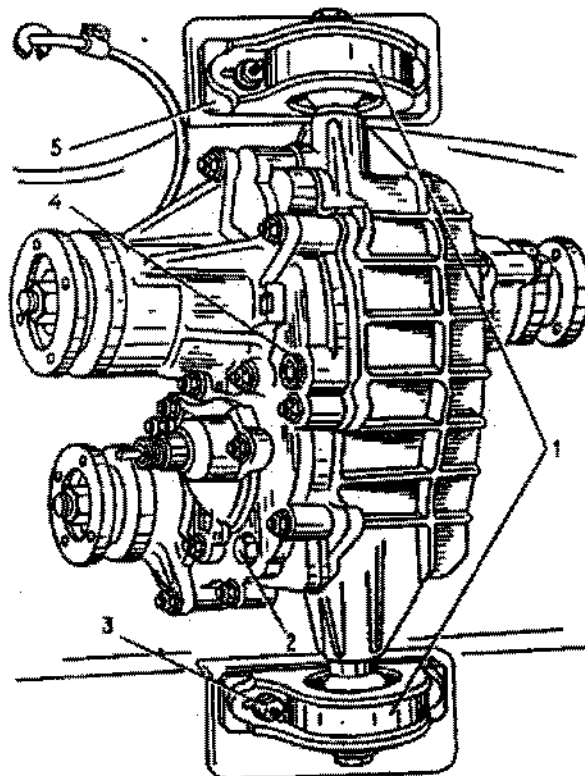
Fig. 3-31. Fixação da caixa de transferência: 1 - suportes da caixa de transferência; 2 - bocal de abastecimento e verificação do nível de óleo; 3 - porca de fixação dos suportes; 4 - bocal de drenagem do óleo lubrificante; 5 - calços de regulagem.
