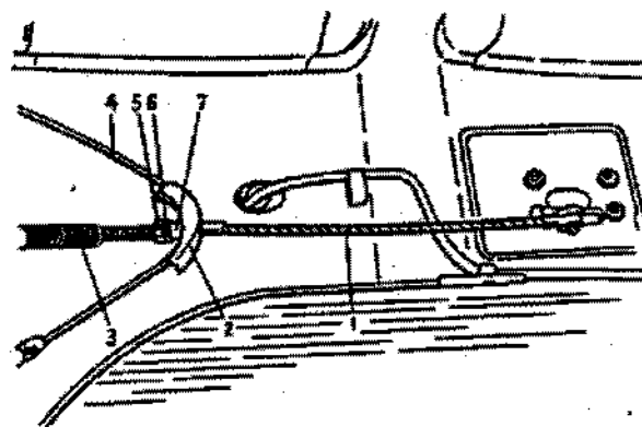
Fig. 6-4. Ajuste do freio de estacionamento: 1 - cabo dianteiro; 2 - equalizador do cabo traseiro; 3 - mola de retorno do cabo traseiro; 4 - cabo traseiro; 5 - contraporca; 6 - porca de ajuste; 7 - espaçador.
